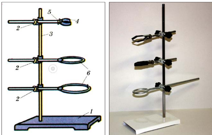
Мал. 10. Лабораторний штатив
