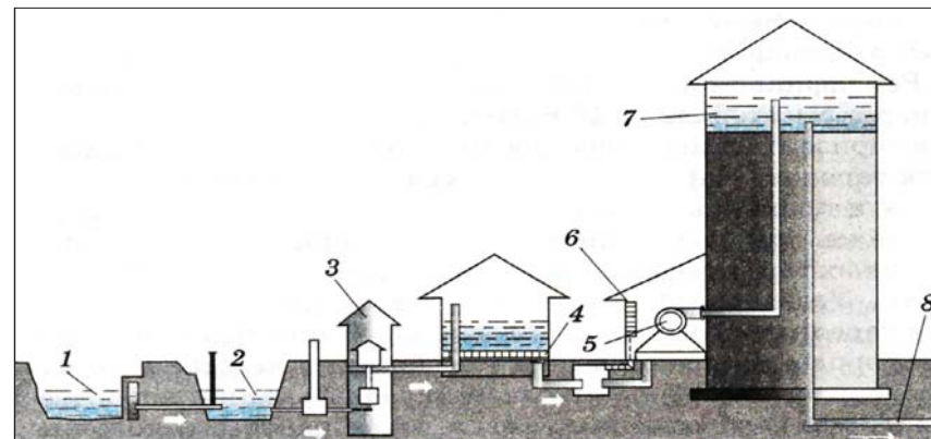
Мал. 55. Схема очищення річкової води на водоочисній станції: 1 – ріка; 2 – басейн для відстоювання води; 3 – колодязь; 4 – фільтр; 5 – насос; 6 – пристрій для хлорування води; 7 – водонапірна башта; 8 – водопровід до міста
