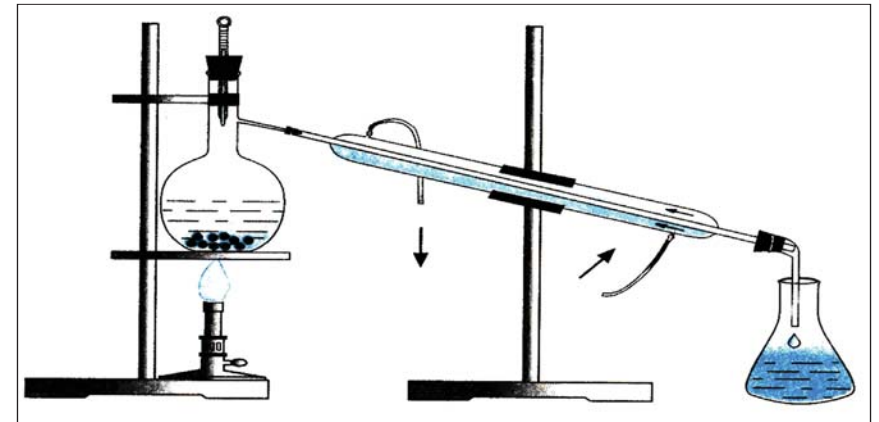
Мал. 21. Прилад для перегонки рідких сумішей
