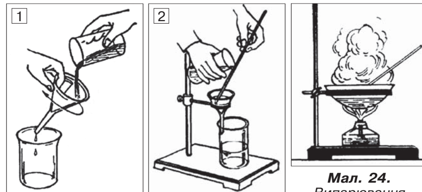
Мал. 23. 1 – змочування фільтра водою; 2 – фільтрування
