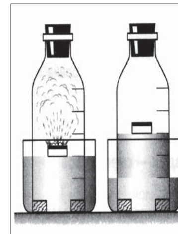
Мал. 39. Визначення об'ємної частки кисню в повітрі
