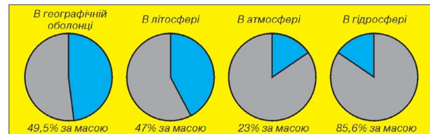
Мал. 38. Діаграма поширеності Оксигену в природі
