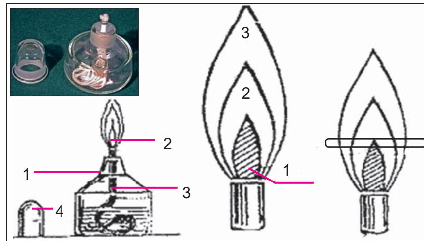
Мал. 11. Спиртівка та полум'я спиртівки
