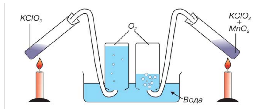
Мал. 43. Прискорення реакції виділення кисню в присутності каталізатора \text{MnO}_2 порівняно з реакцією, де каталізатор відсутній
