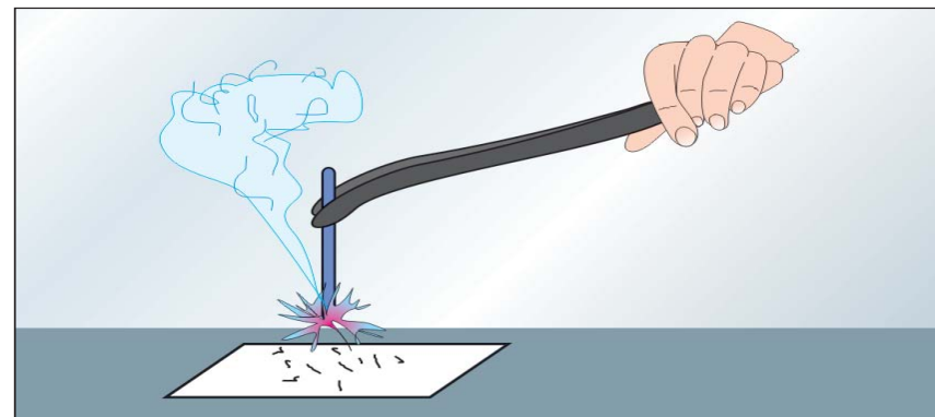
Мал. 44. Горіння магнію
