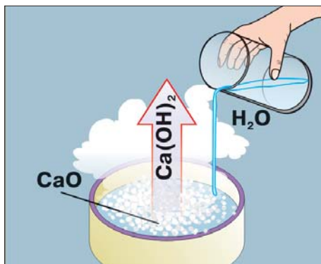
Мал. 53. Взаємодія негашеного вапна \text{CaO} з водою
