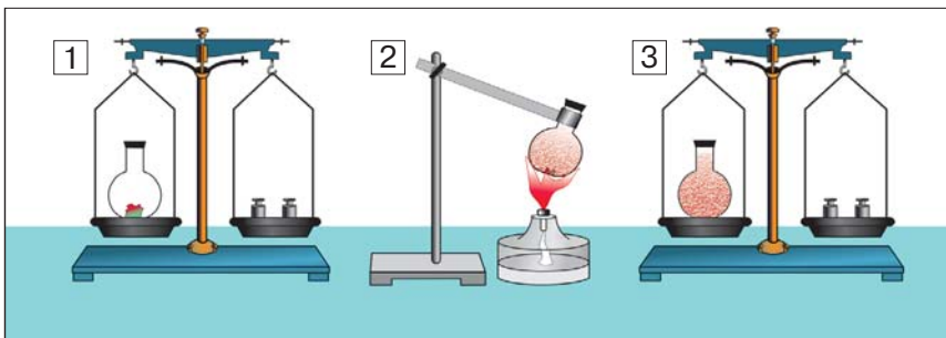
Мал. 40. Дослід, що підтверджує закон збереження маси речовини в хімічних реакціях: 1 – зважування до реакції; 2 – взаємодія речовин при нагріванні; 3 – зважування після реакції
