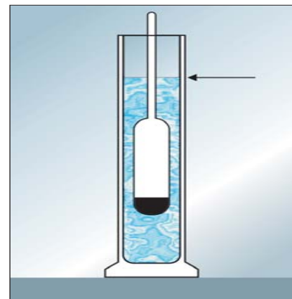
Мал. 15. Визначення густини рідини ареометром
