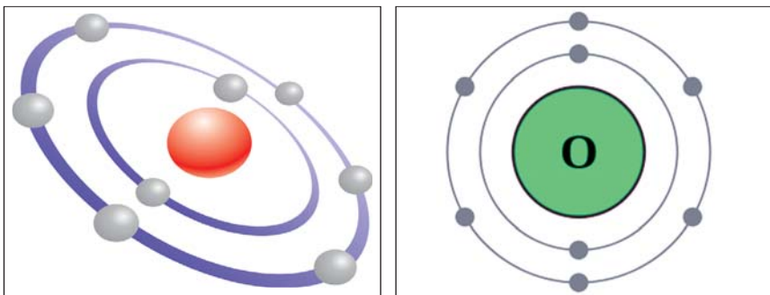
Мал. 29. Моделі будови атома Оксигену
