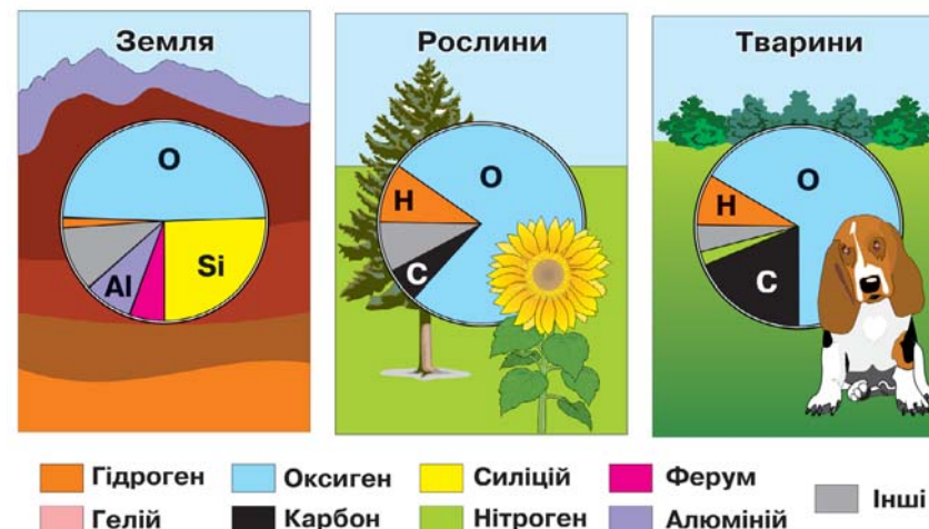
Мал. 48. Вміст елементів у земній корі та організмах тварин і рослин різний
