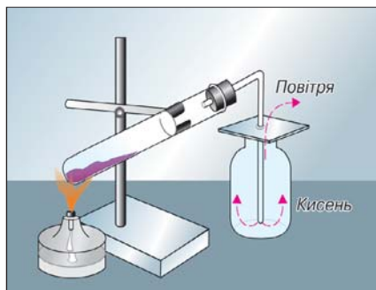
Мал. 41. Добування кисню і збирання його в банку шляхом витіснення повітря
